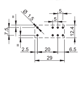
Vista lato rame Lunghezza pin 3.5 mm per circuito stampato Lunghezza pin 5.3 mm per zoccolo o montaggio su circuito stampato Vedere codificazione
