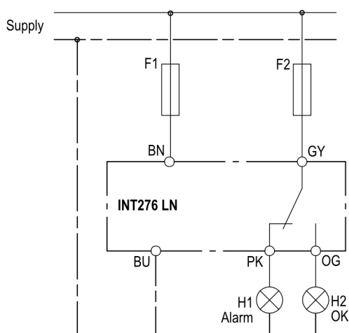
Anschluss-Schaltbild
